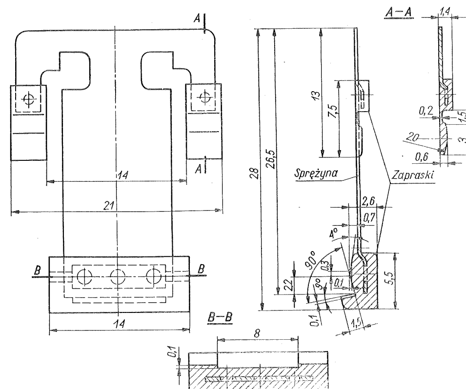
Rys. 31 Sprężyna łożyskowa kompletna przełącznika C11
