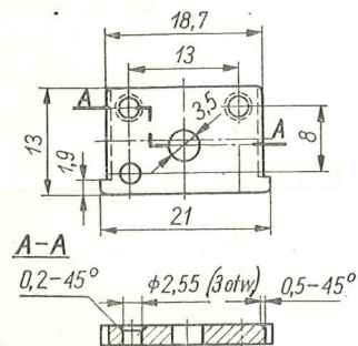
Rys. 34 Podkładka metalowa dolna układu zestyków przełącznika C11
