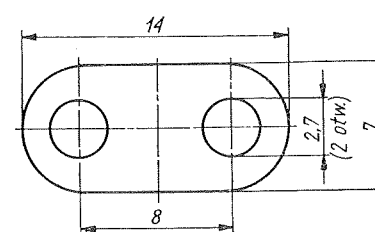
Rys. 32 Podkładka sprężyny łożyskowej kompletny przełącznika C11
