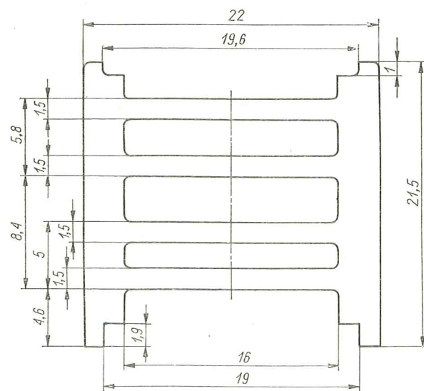
Rys. 28d Drabinka układów zestyków przełącznika C11 czteroszczeblowa o niesymetrycznym rozłożeniu szczebli
