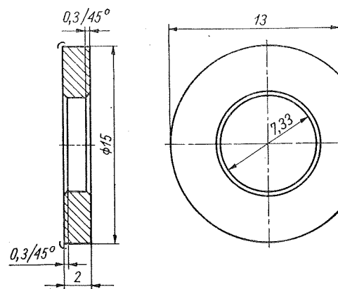
Rys. 30 Nabiegunnik przełącznika C11
