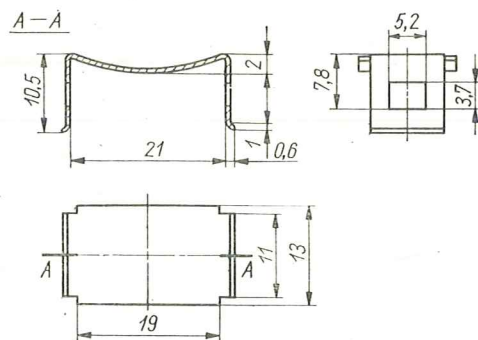
Rys. 36 Sprężyna spinająca układ zestyków przełącznika C11
