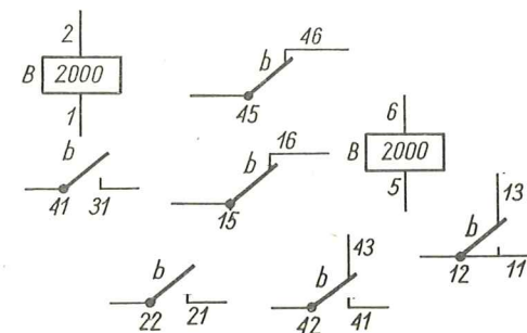
Rys. 5 Oznaczenia schematowe sprężyn stykowych w zestykach i zwojnic cewki przekaźnika C11
