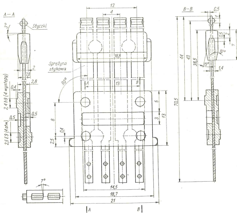
Rys. 24 Zespół sprężyn stykowych stałych ze stycznymi z dwóch stron sprężyn stykowych przekładników C11
