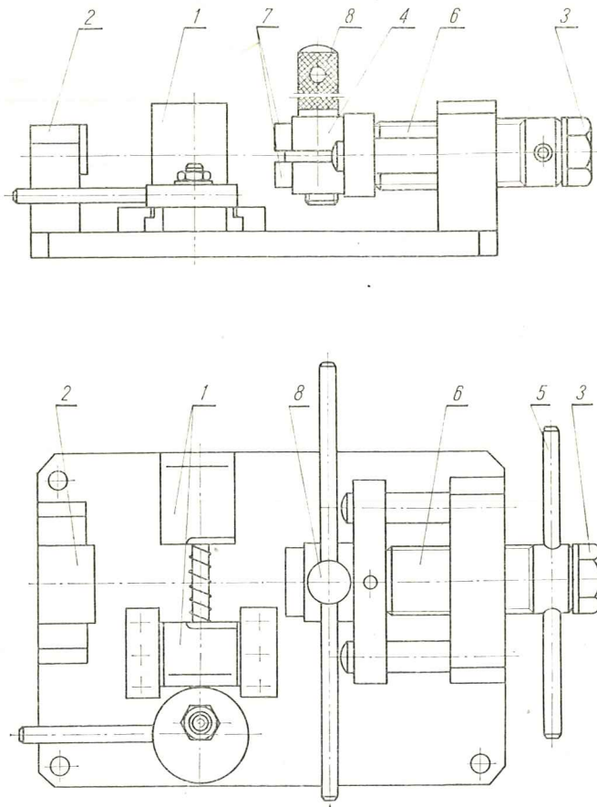
Rys. 61 Przyrząd do wciskania i ściągania nabiegownika z rdzenia korpusu kompletnego przekaźnika C11
