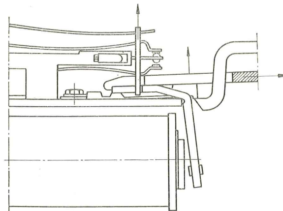
Rys. 60 Sposób zdejmowania kotwicy kompletnej z przełącznika C11
