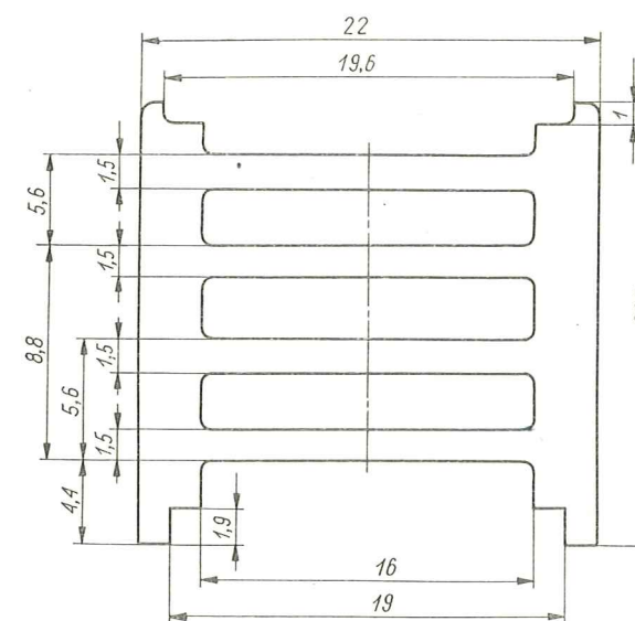
Rys. 28b Drabinka układów zestyków przełącznika C11 czteroszczebłowa
