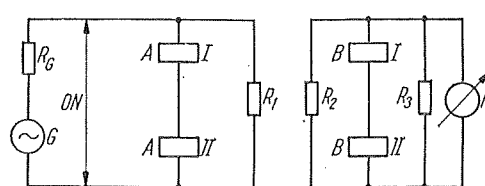
Rys. 44 Schemat układu do pomiaru tłumienności przesłuchu przekaźników C11
