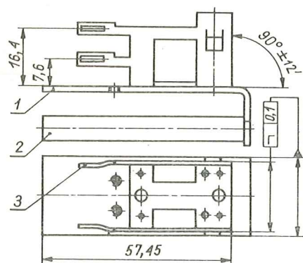
Rys. 11 Korpus kompletny przekaźnika C11 dla 6-8 zestyków
