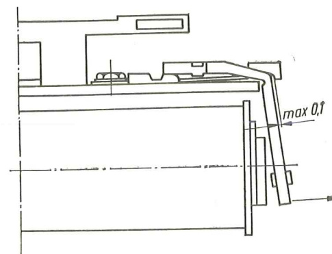
Rys. 53 Miejsce pomiaru szczeliny między zaczepem zapraski sprężyny łożyskowej a kotwicą kompletną
