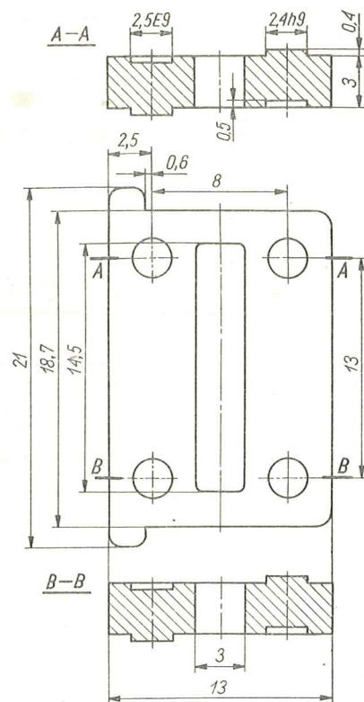
Rys. 26 Przekładka izolacyjna układów zestyków przełączników C11
