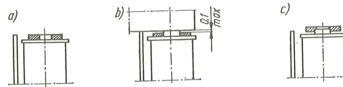
Rys. 54 Położenie powierzchni czołowej nabiegownika na rdzeniu korpusu kompletnej przełącznika C11
