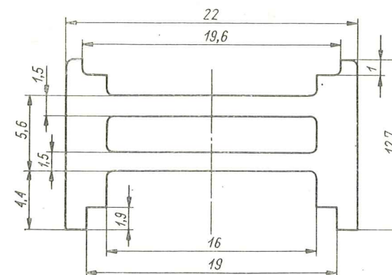
Rys. 28a Drabinka układów zestyków przełącznika C11 dwuszczebłowa
