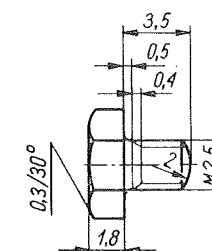
Rys. 33 Śruba mocująca sprężynę łożyskową kompletną przełącznika C11
