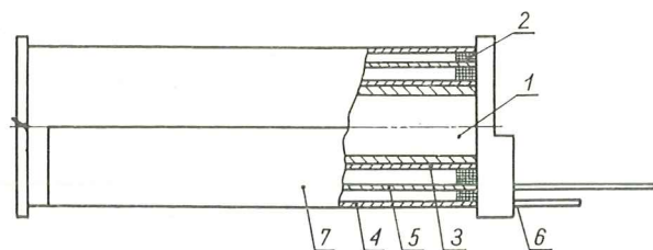
Rys. 17 Konstrukcja cewki przełącznika C11
