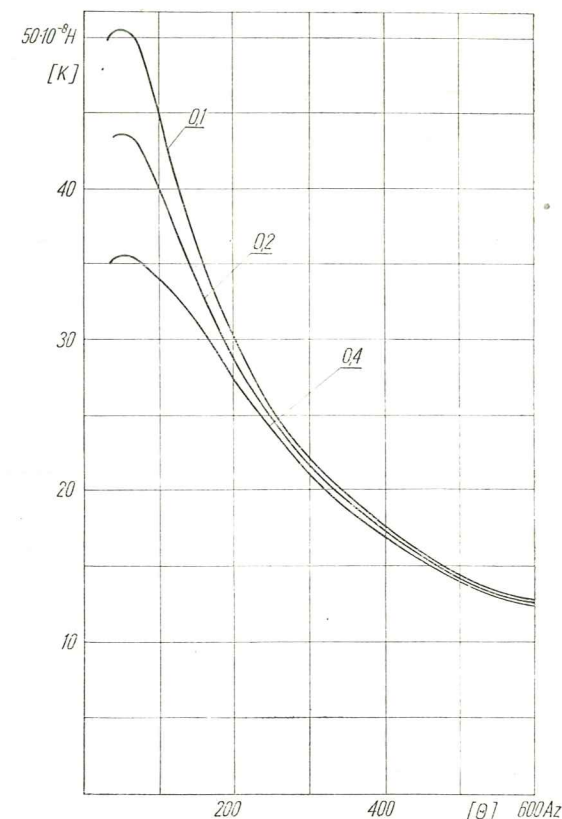
Rys. 46 Wykres współczynnika k , określającego indukcyjność przełącznika C11 w funkcji siły magnetomotorycznej, wytwarzanej przez zwojnicę cewki przełącznika, przy kotwicy przyciągniętej i grubościach płytek niemagnetycznych 0,1, 0,2 i 0,4 mm
