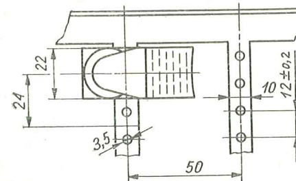
Rys. 37 Sposób mocowania przełączników C11 do podstawy przełącznikowej
