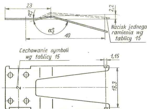
Rys. 27 Sprężyna zwrotna układu zestyków przełącznika C11
