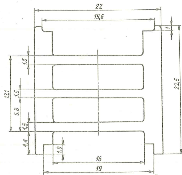
Rys. 28c Drabinka układów zestyków przełącznika C11 trzyszczeblowa
