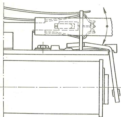
Rys. 55 Sposób gięcia ramion wspornika korpusu kompletnego przełącznika C11
