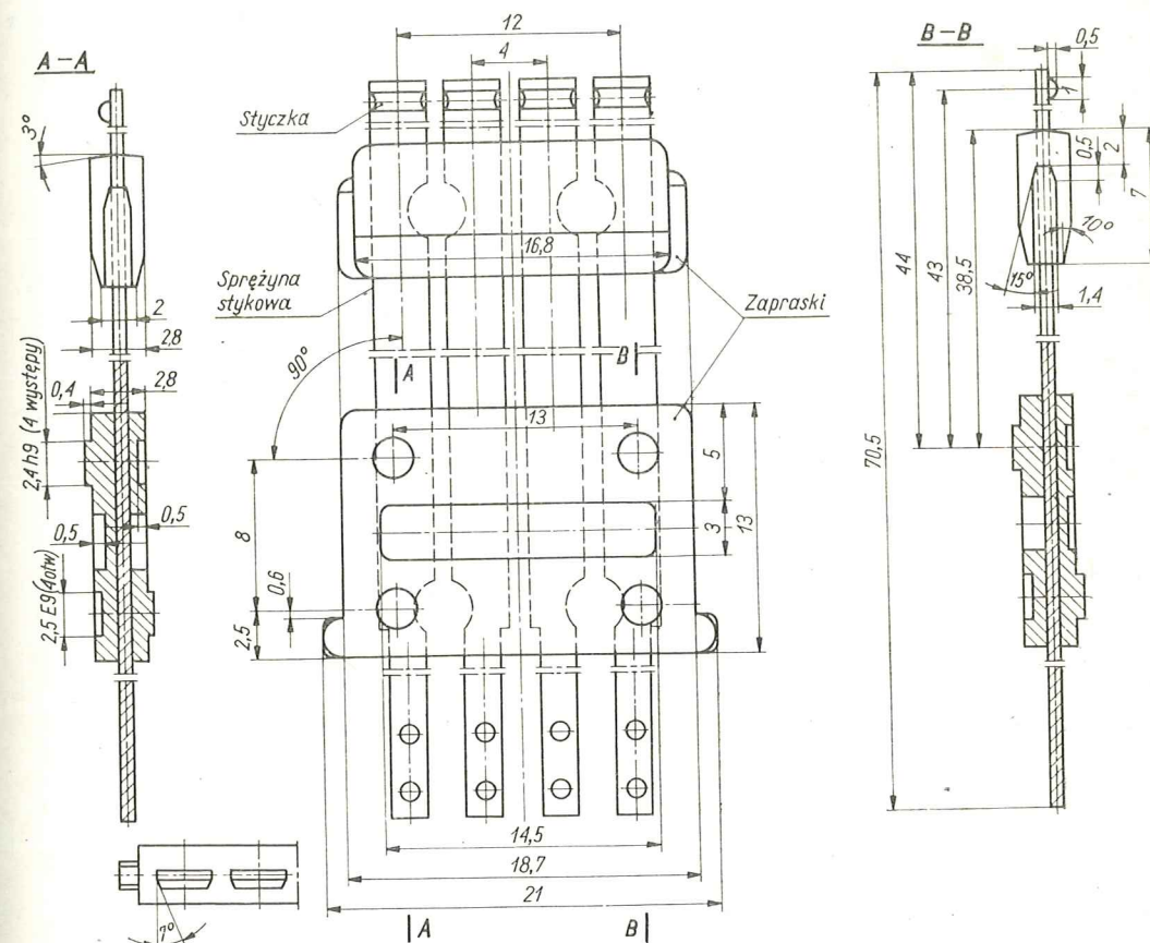
Rys. 25 Zespół sprężyn stykowych stałych ze stycznymi z jednej strony sprężyn stykowych przekładników C11
