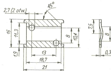
Rys. 35 Podkładka metalowa górna układu zestyków przełącznika C11
