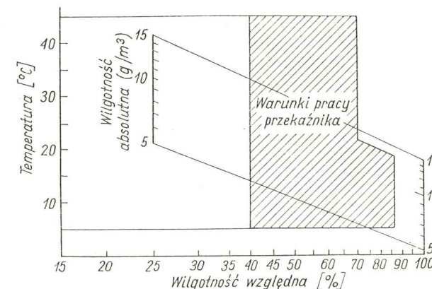
Rys. 39 Graniczne warunki atmosferyczne pracy przełącznika C11 o kategorii klimatycznej 576 wg PN-60/T-04550
