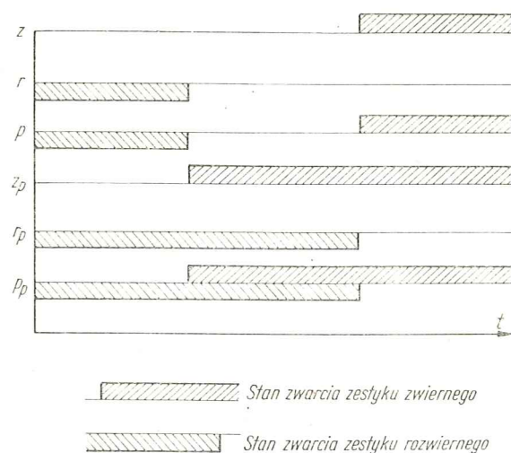
Rys. 40 Przebieg działania zestyków przełączników C11 z — zwierne, r — rozwierne, p — przełączne, z_p — zwierne przesunięte, r_p — rozwierne przesunięte, p_p — przełączne bezprzerwowe
