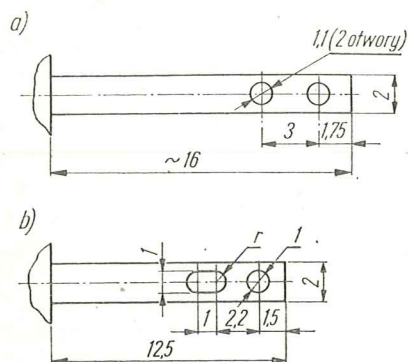
Rys. 41 Kształt końcówek lutowniczych przełącznika C11 a — sprężyn stykowych, b — końcówek cewki
