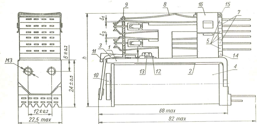
Rys. 2 Konstrukcja przełącznika C11
