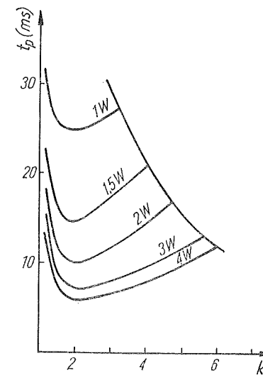
Rys. 43 Wykres czasów przyciągania przekaźnika C11 w funkcji współczynnika zapasu ( k_2 ) dla różnych wartości mocy traconej w zwojnicy
