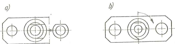
Rys. 62 Sposób mocowania nabiegownika w tulei prowadzącej
